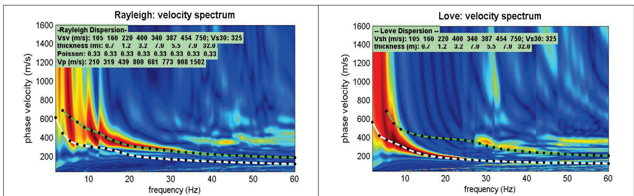
Fig. 6 – Spettri di velocità con curva di dispersione da analisi congiunta Onde di Rayleigh + Onde di Love Spettro Rayleigh (a sinistra) e Spettro di Love (a destra)
