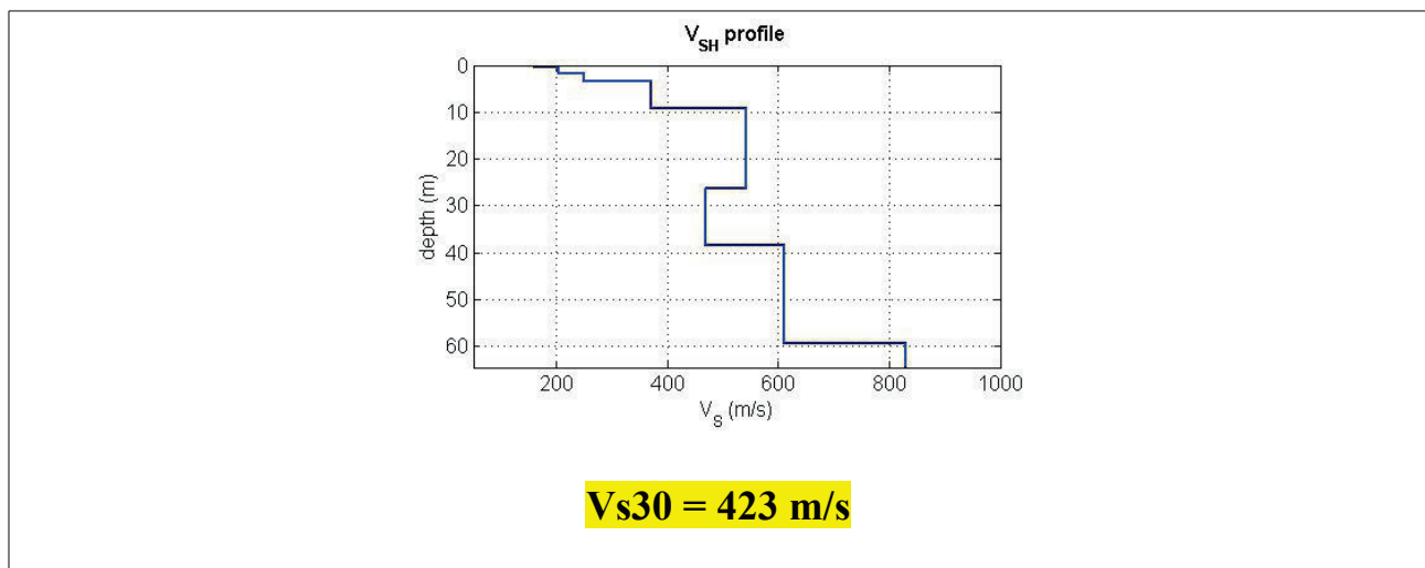
Fig. 2 – Sismostratigrafia associata al modello estrapolato
