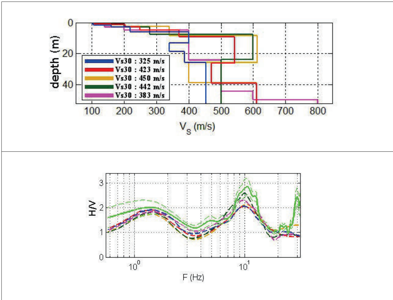
Fig. 8 – Sopra: alcuni dei possibili modelli sismostratigrafici estrapolati da sola indagine HVSR Sotto: Curve H/V dei modelli ottenuti (verde = sito in esame; altri colori = curve modelli da sola indagine HVSR)
