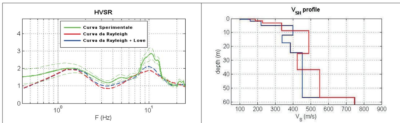
Fig. 7 – Confronto delle curve H/V (a sinistra) e delle sismostratigrafie (a destra) derivanti dalle precedenti analisi.
