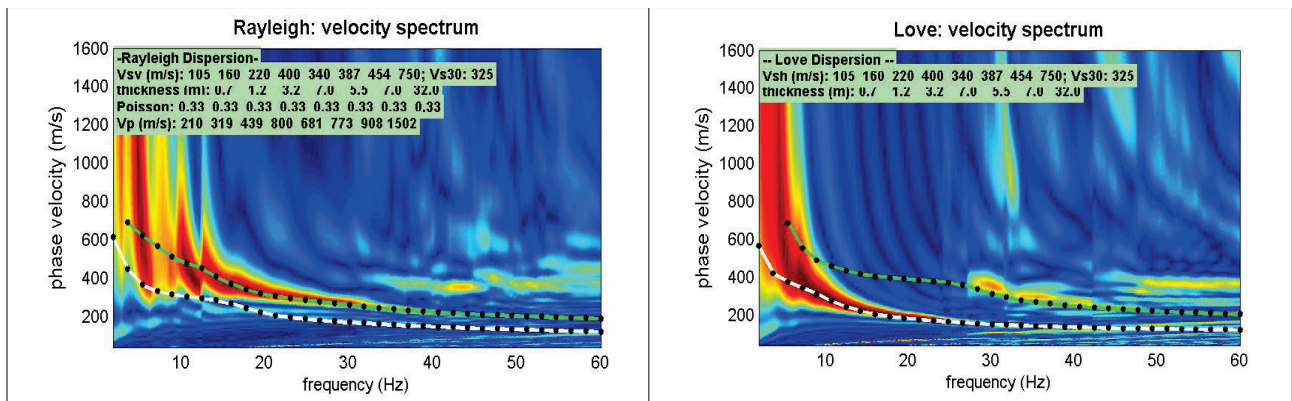
Fig. 3 – Spettri di velocità con curve di dispersione: Onde di Rayleigh (a sinistra) e Onde di Love (a destra)
