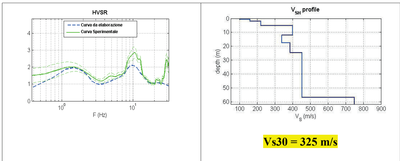
Fig. 4 – Curve H/V (a sinistra) e sismostratigrafia associata al modello estrapolato (a destra)
