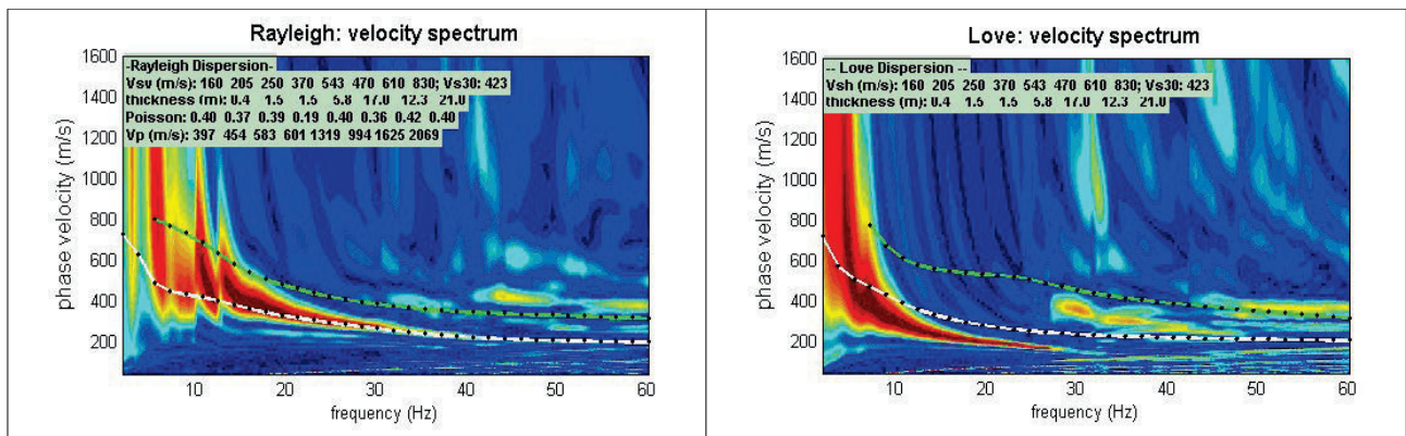
Fig. 5 – Spettri di velocità con curva di dispersione da analisi in sole Onde di Rayleigh: Spettro Rayleigh (a sinistra) e Spettro Love (a destra)
