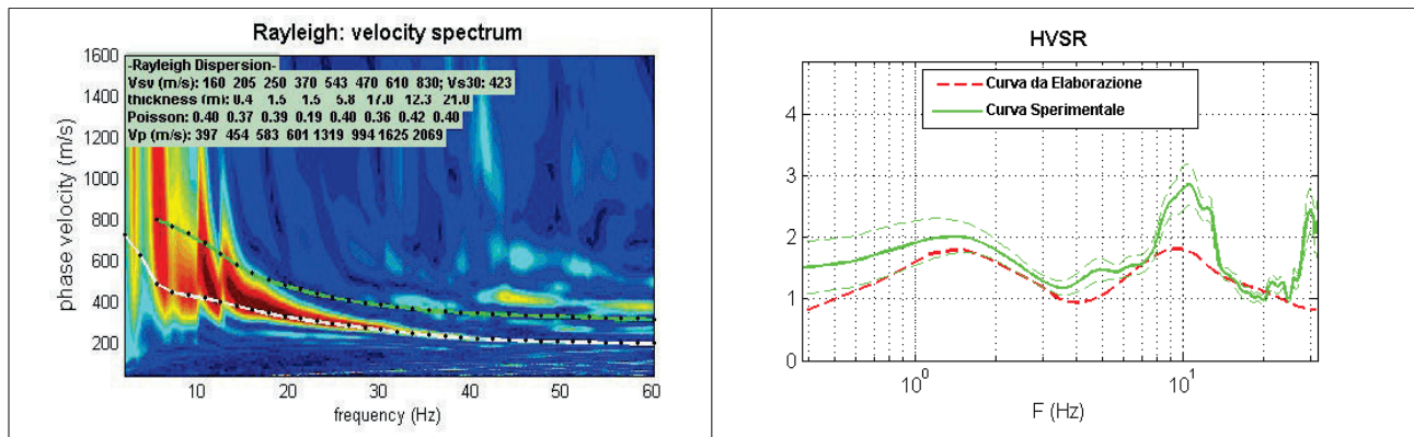
Fig. 1 – Spettro di velocità con curva di dispersione (a sinistra) e curve H/V (a destra)
